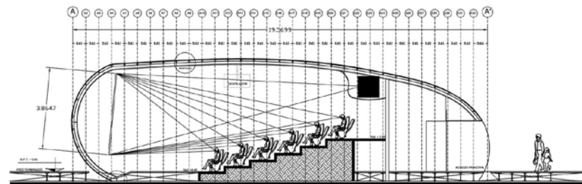
Corte Longitudinal ARQ-HPE-02
